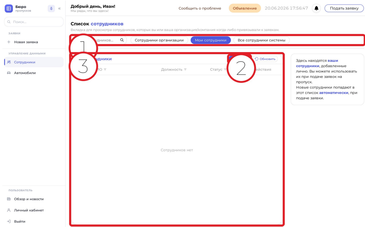
Рисунок 8 — Раздел «Сотрудники»
