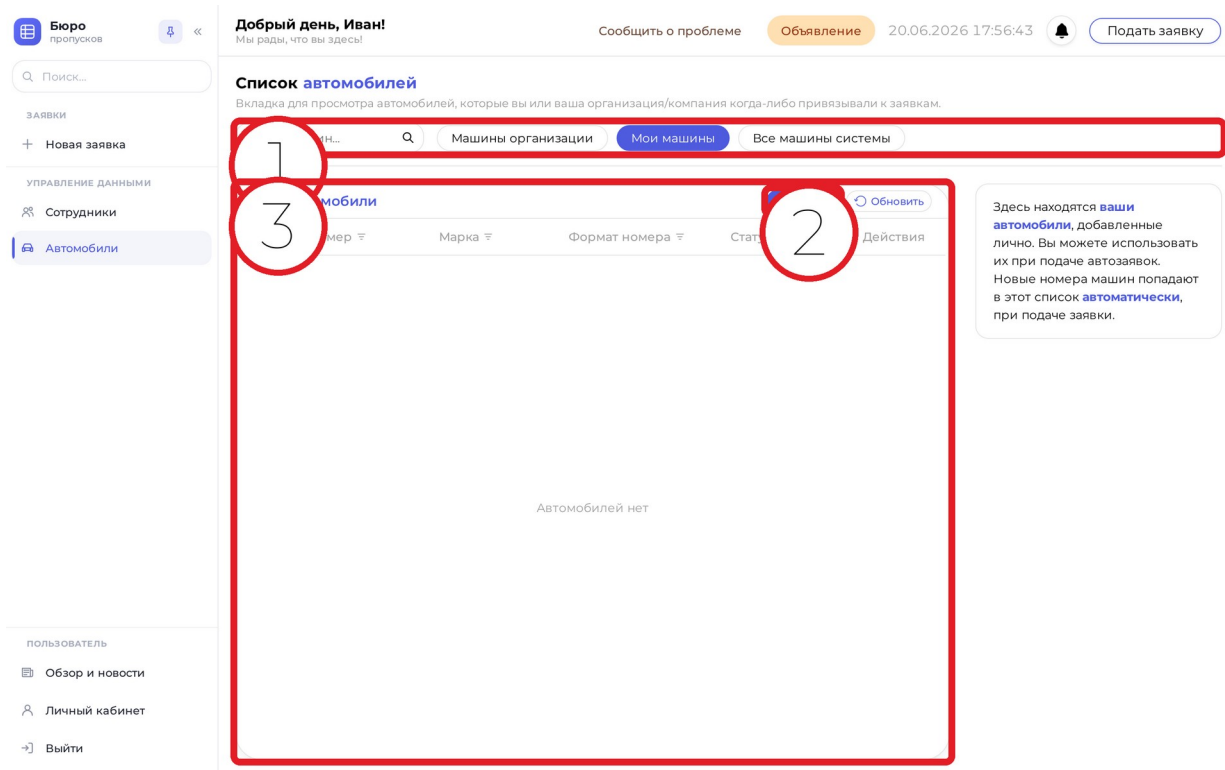
Рисунок 6 — Раздел «Автомобили»
