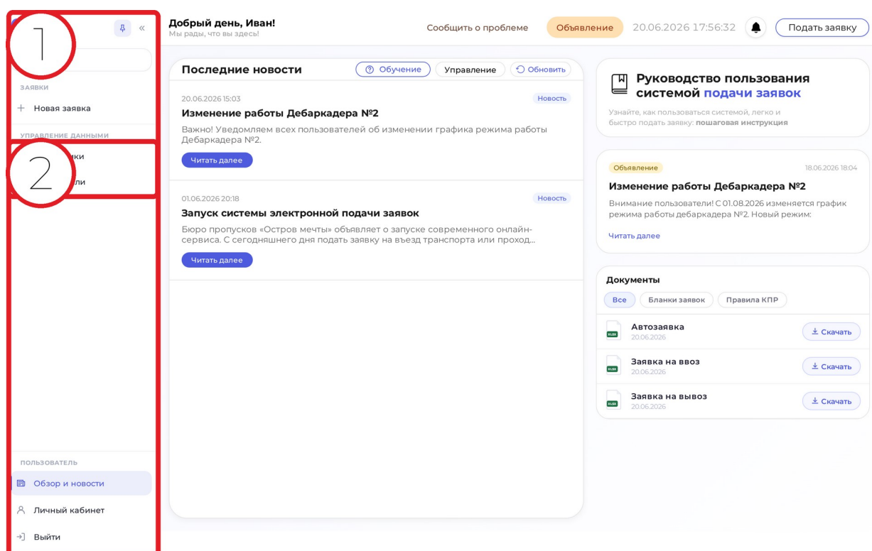
Рисунок 3 — Панель навигации
