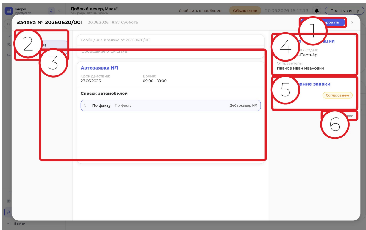
Рисунок 17 — Карточка заявки
